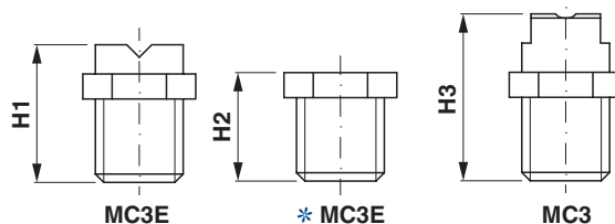
Dimensioni mm Dimensions mm Dimensions mm Abmessungen mm Dimensiones mm
