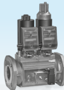
VCS..F avec indicateur de position et pressostat
